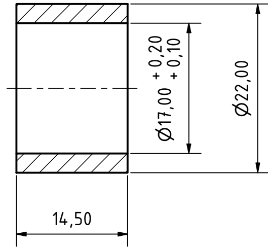
A-A ( 2 : 1 )
